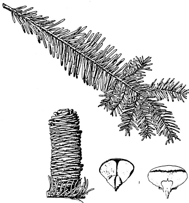
Abies grandis Grand fir ABGR
