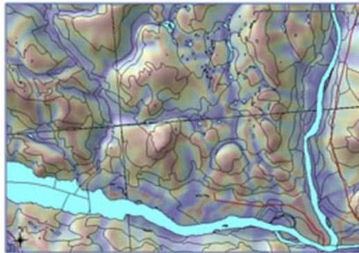
Close up of the area shown in (D)
