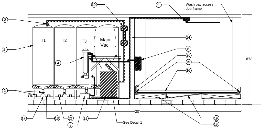
Elevation
